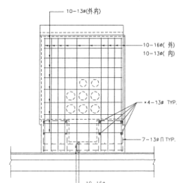
車道側配筋図
