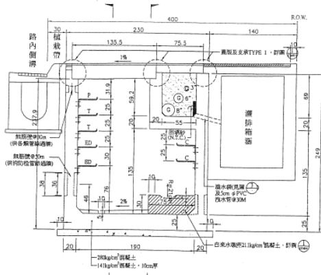
支管共同管道 TYPE I 標準段斷面圖
