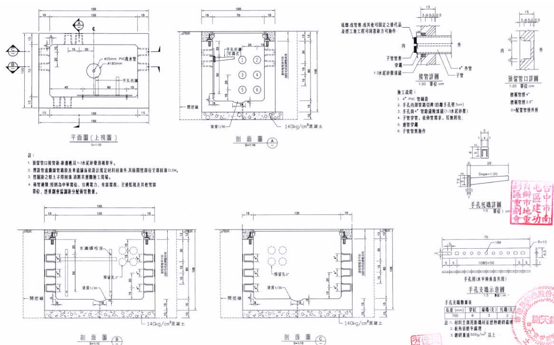
振興路以南區段徵收共同管道斷面圖
