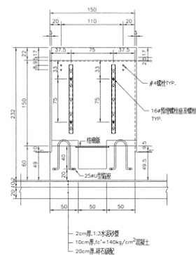
民地側便面圖
