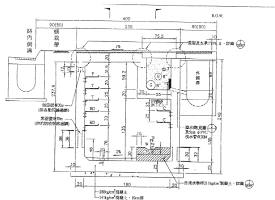
支管共同管道 TYPE I 箱涵段斷面圖
