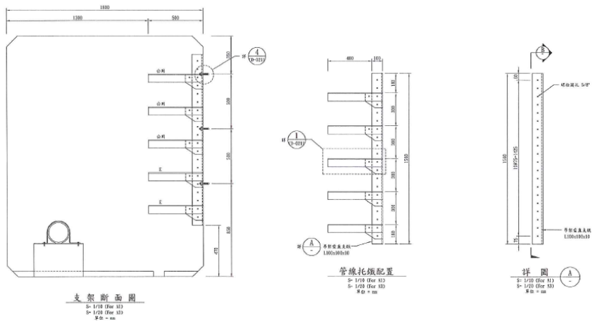
共同管道支架型式規格材料表(支架配置間距10m, 單位)
