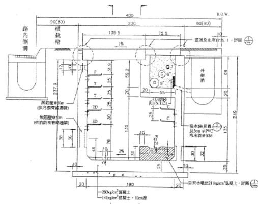
支管共同管道 TYPE I 標準段斷面圖
