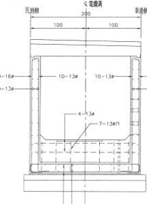
横断面配筋图
