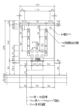
車道側側面圖
