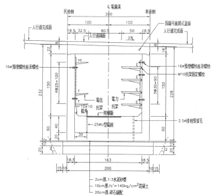
電力連接分枝部橫斷面圖
