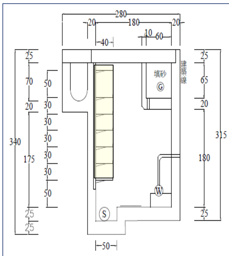
振興路以南區段徵收共同管道斷面圖
