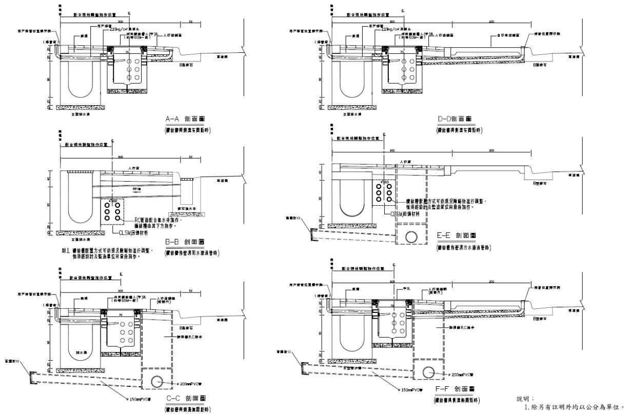
中科經貿自辦市地重劃共同管道斷面圖
