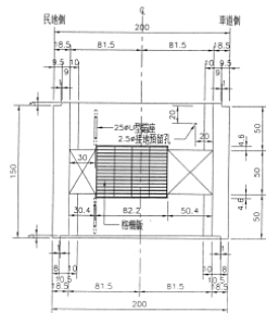
平面圖(蓋版打開)
