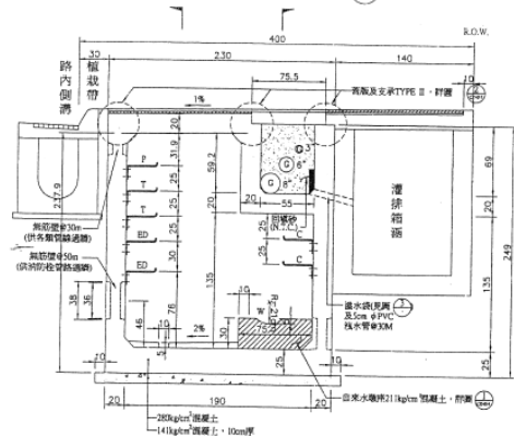
支管共同管道 TYPE I 箱涵段斷面圖
