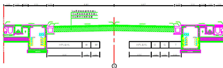
廊子地區區段徵收共同管道斷面圖
