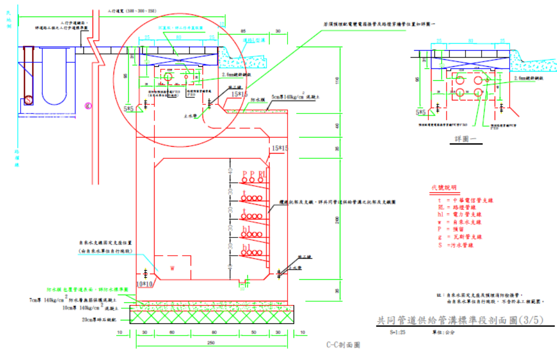
廊子地區區段徵收共同管道斷面圖
